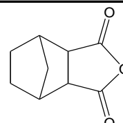
【HNA】
