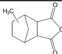
【MeHNA】
